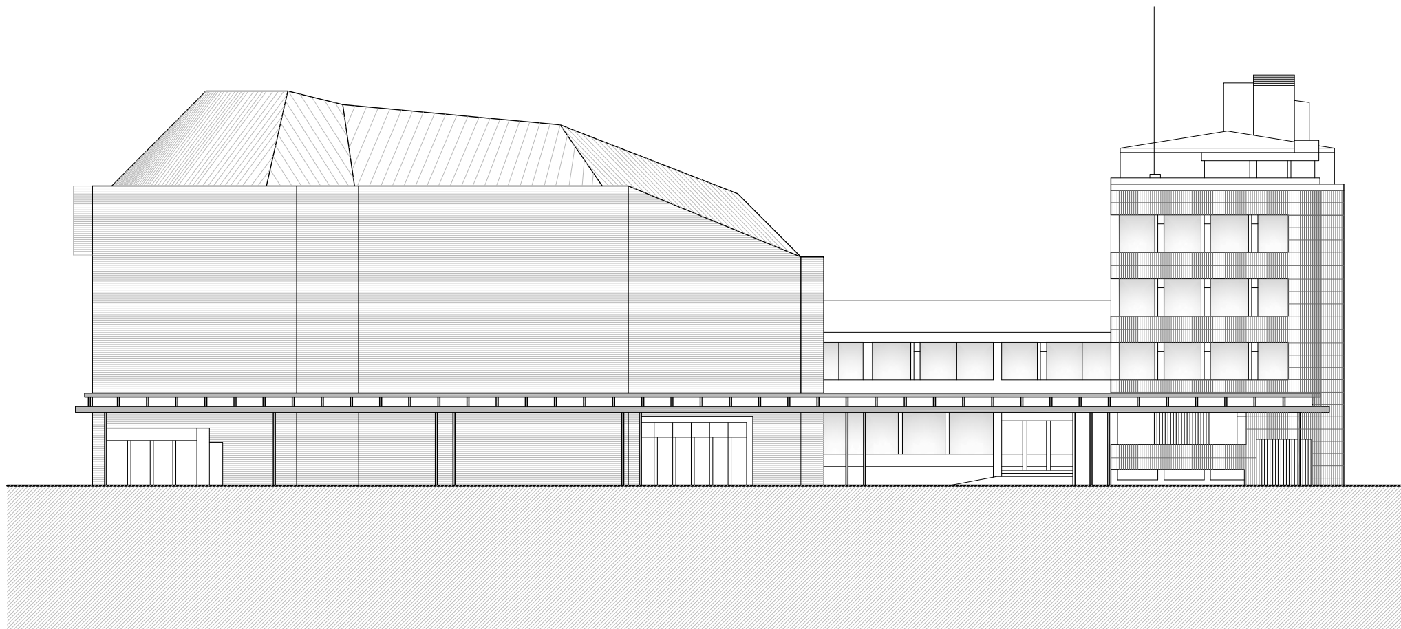
Alçat Sud
