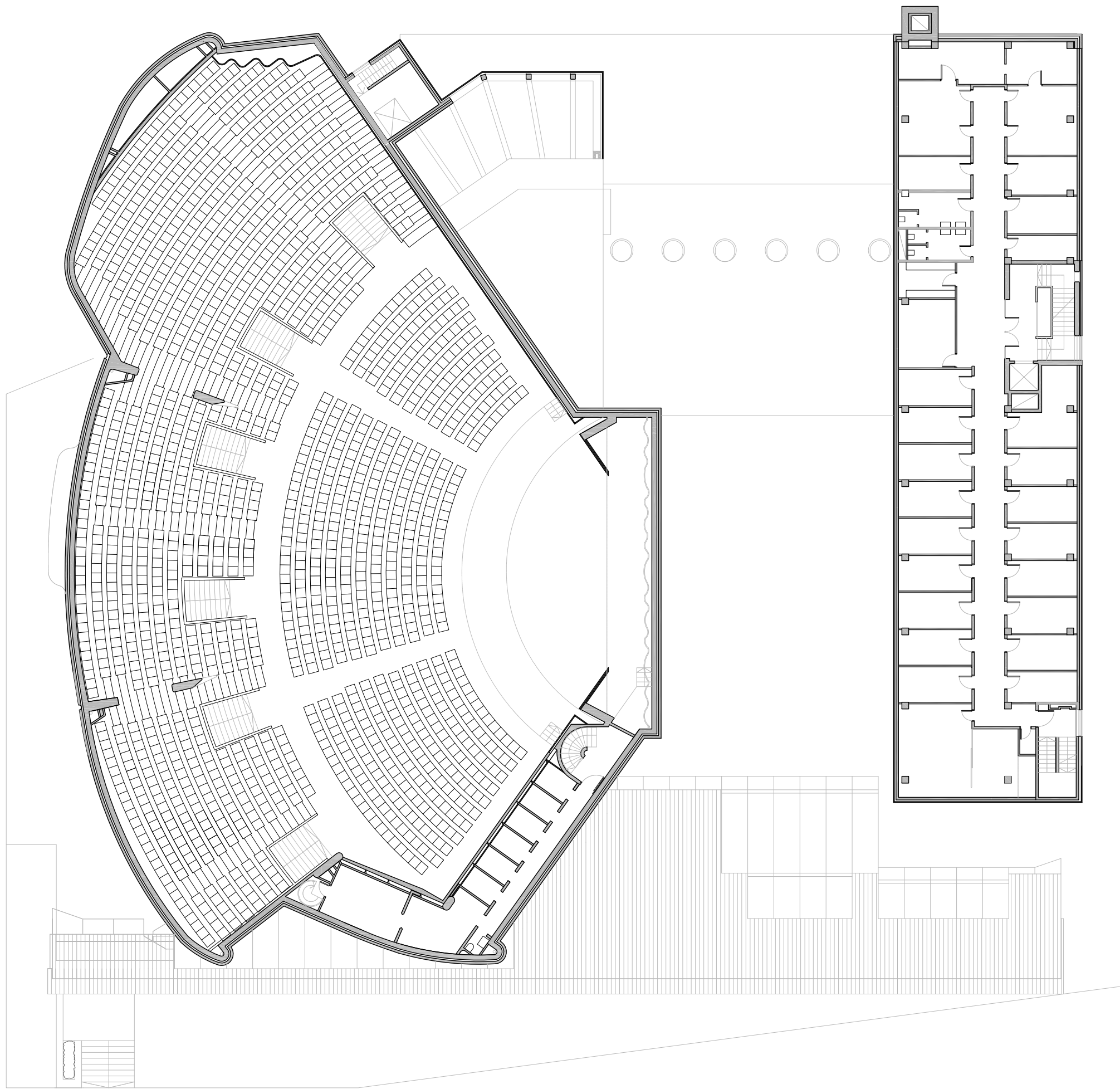
Planta Segona
