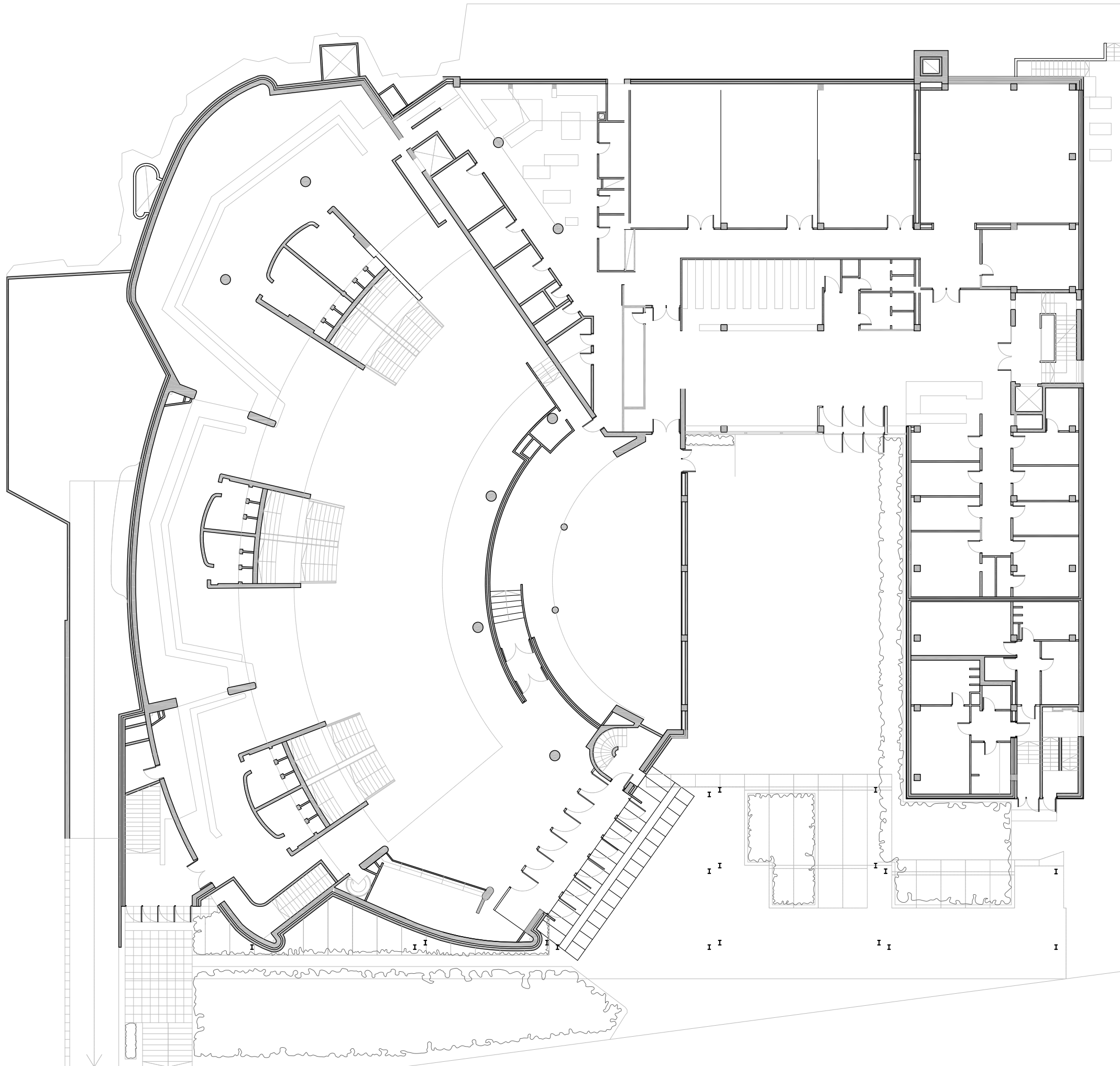
Planta Baja
