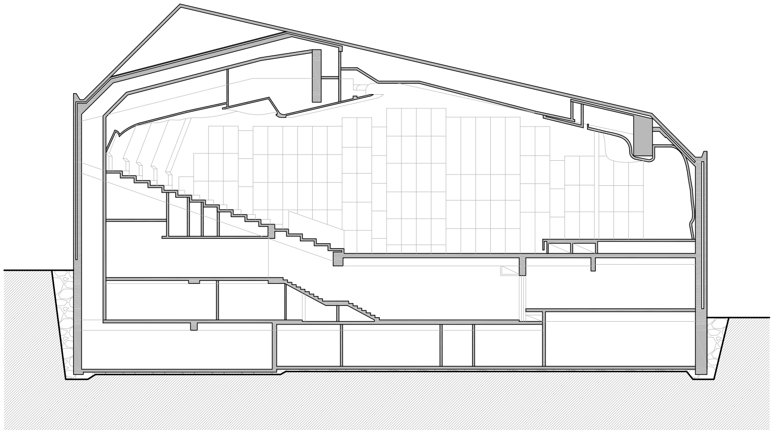
Secció a-a'
