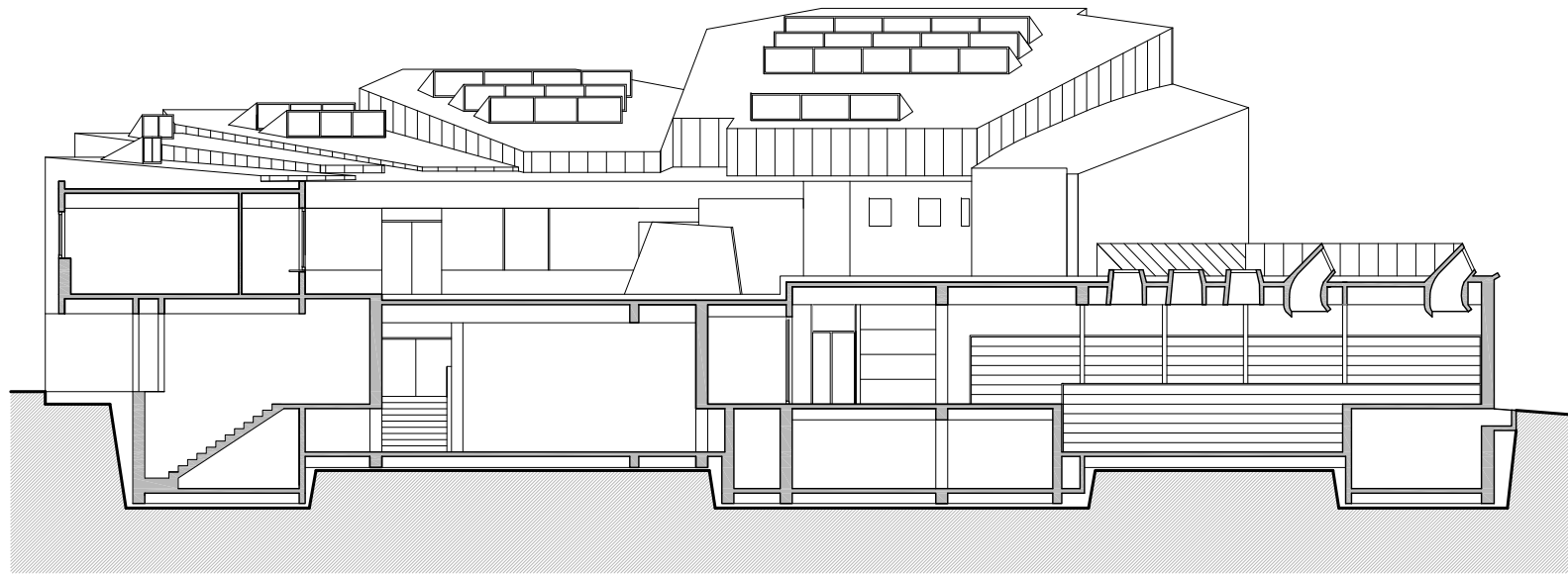
Secció b-b'
