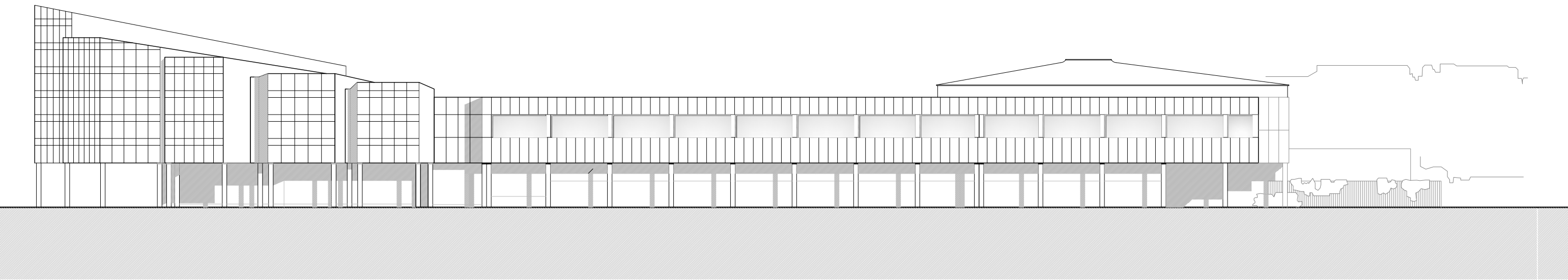
Alçat Oest
