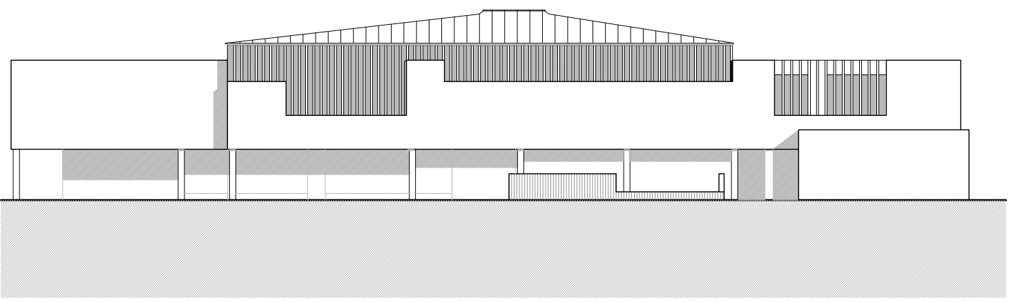
Alçat Sud
