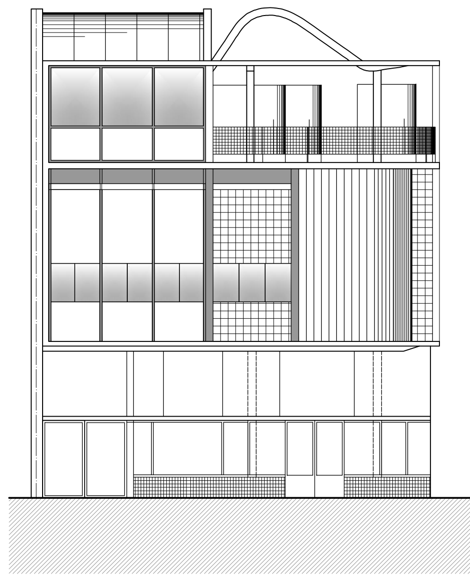
Alçat Nord
