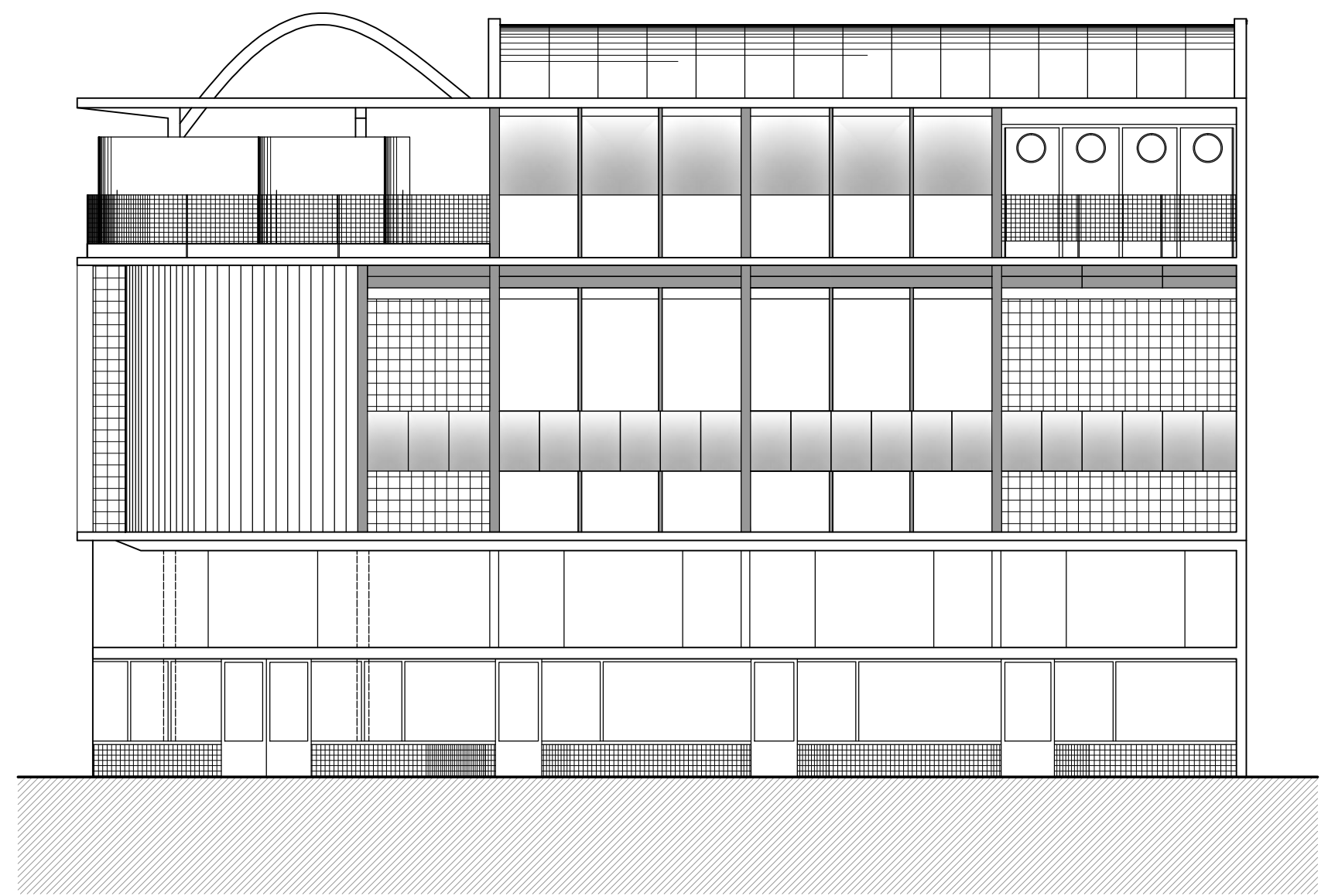
Alçat Oest
