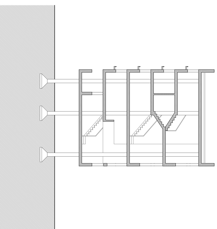
Secció C-C'
