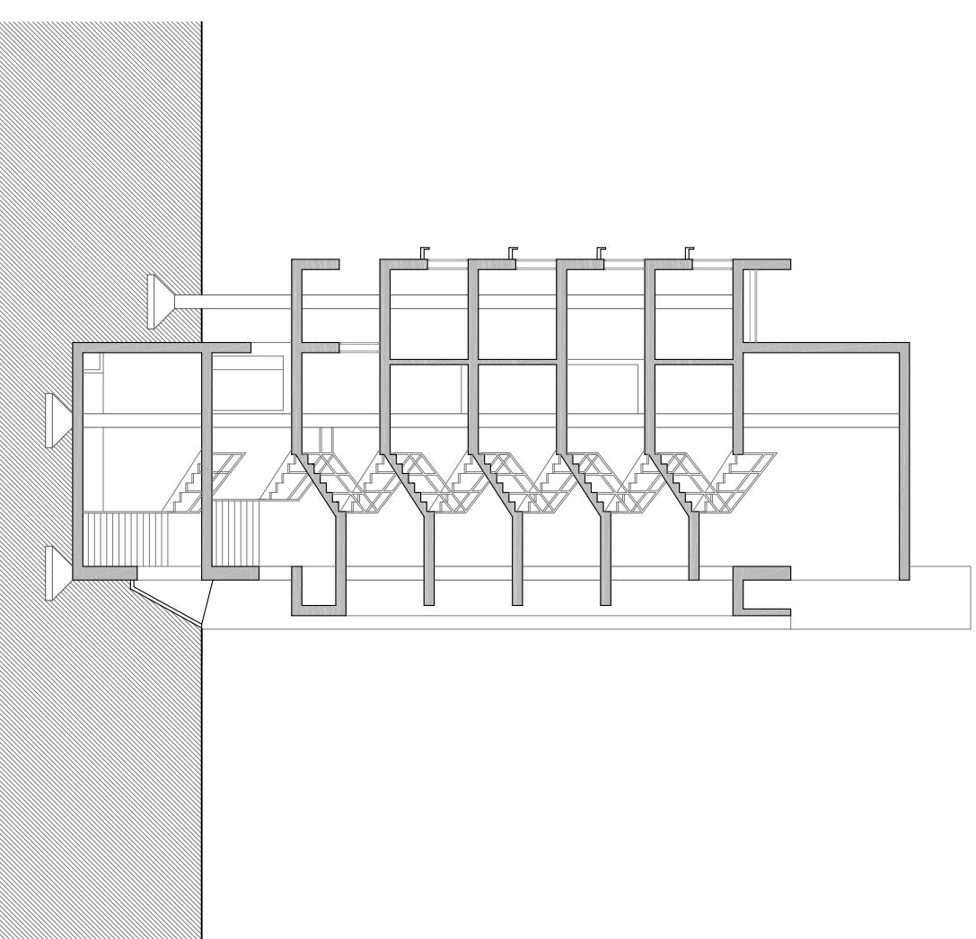
Secció D-D'
