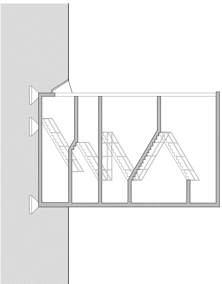
Secció A-A'
