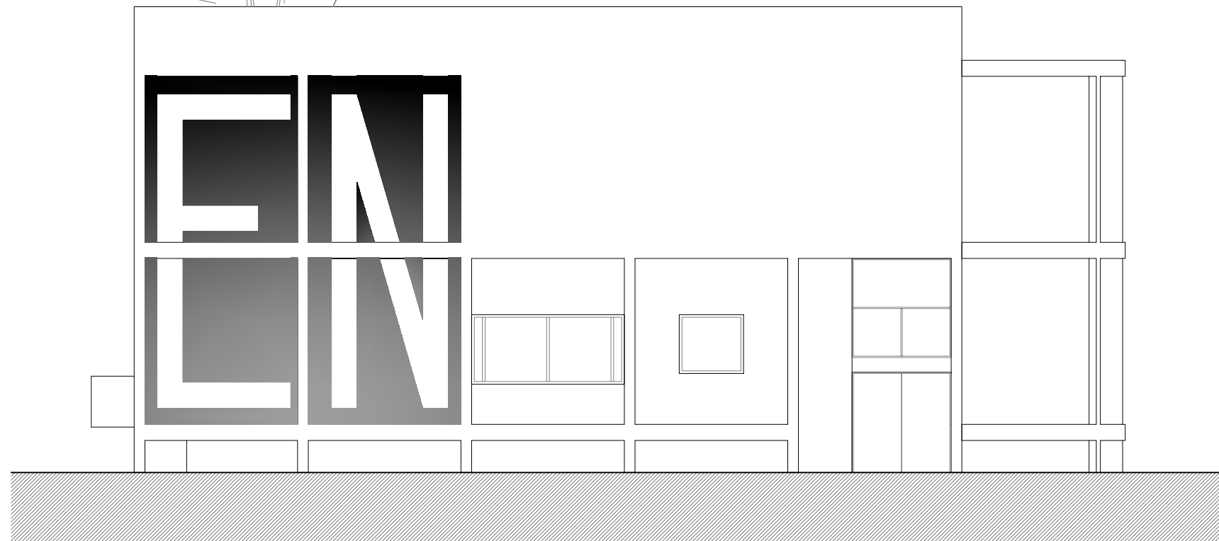
Alçat Oest
