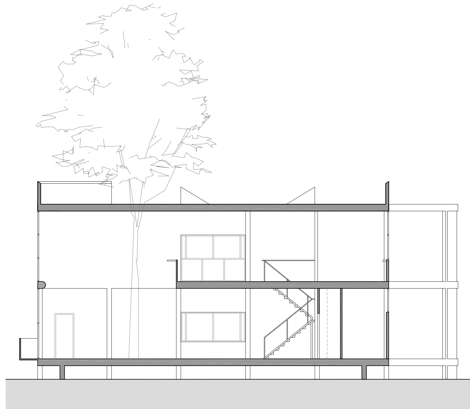
Alçat-Secció
