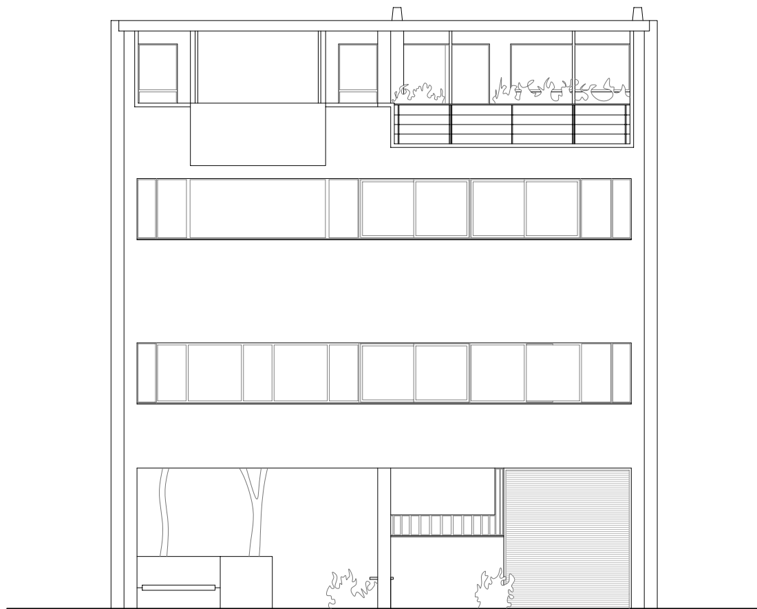
Alçat principal(a carrer)
