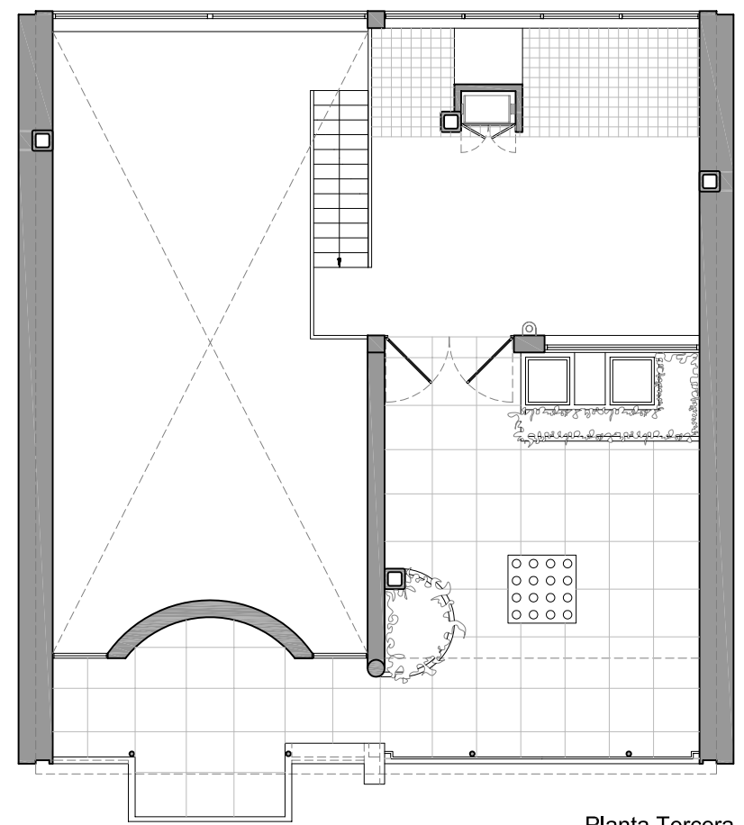
Planta Tercera
