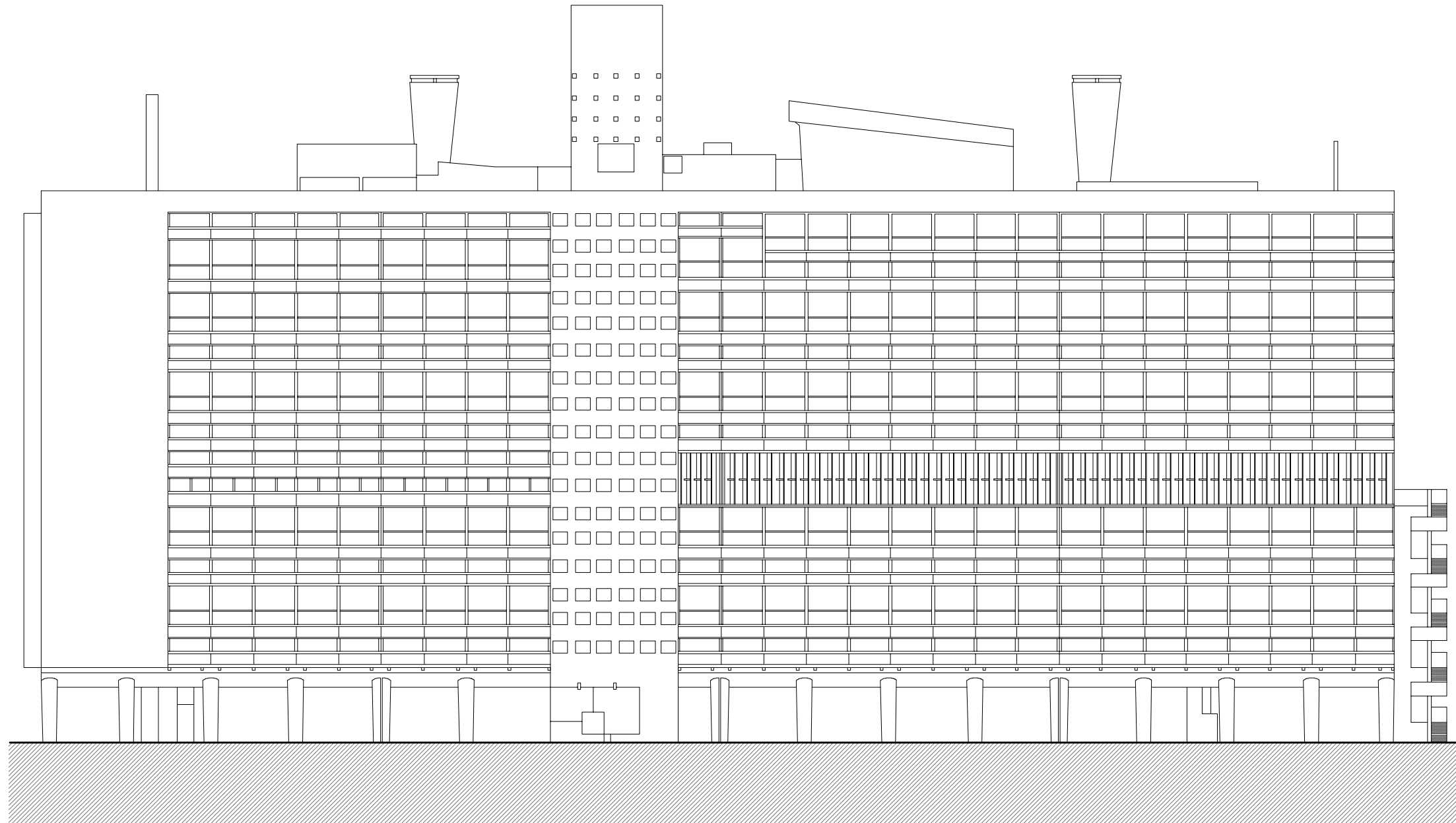
Alçat Est
