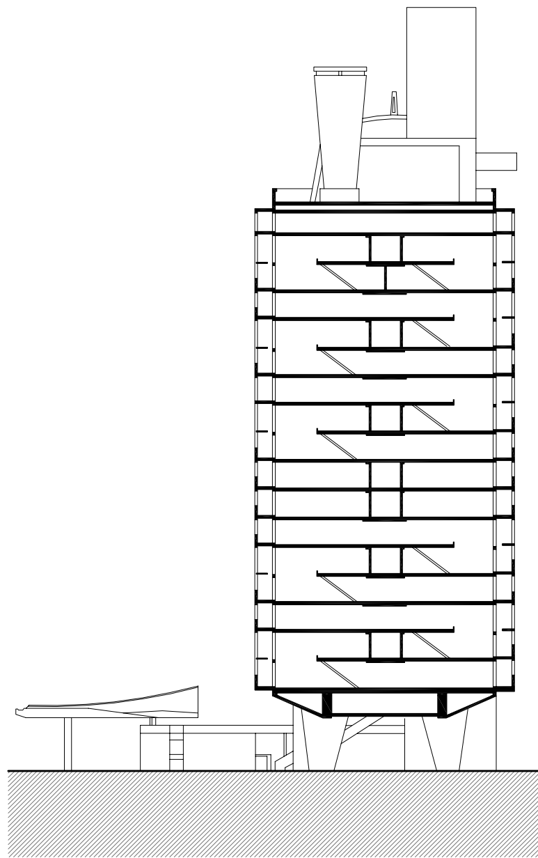
Secció Transversal
