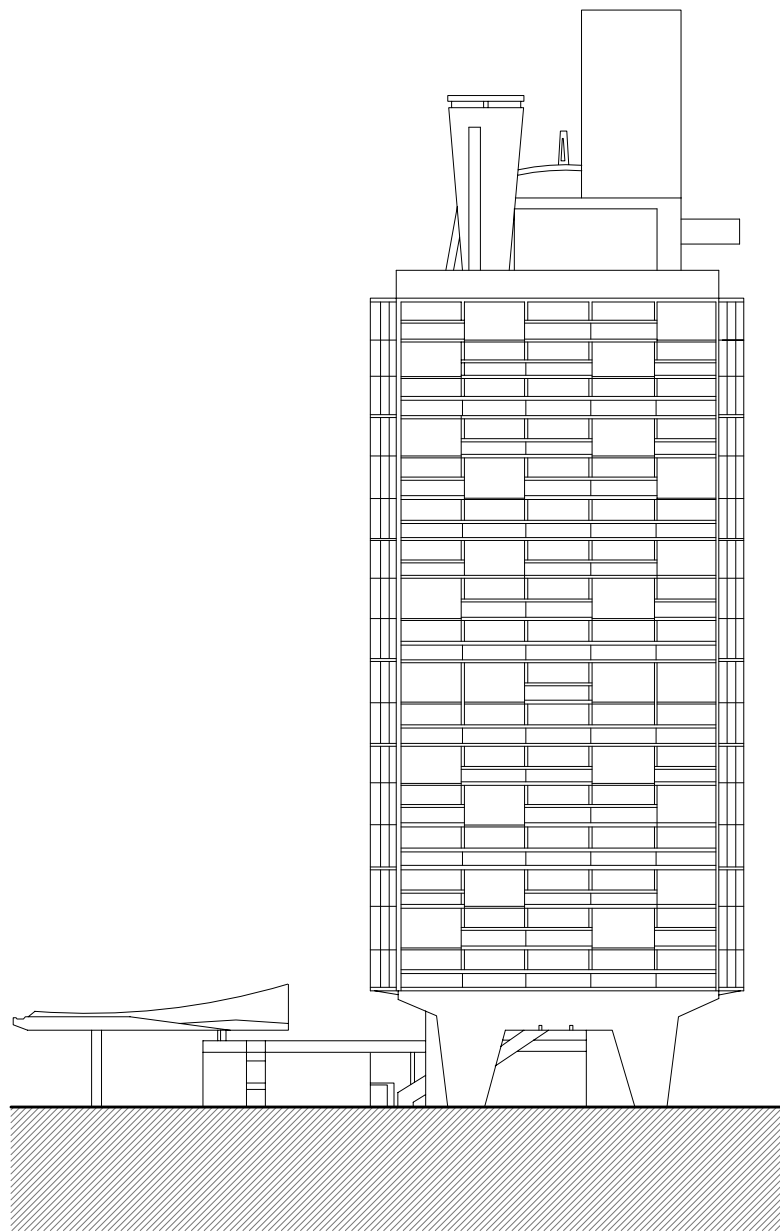
Alçat Sud
