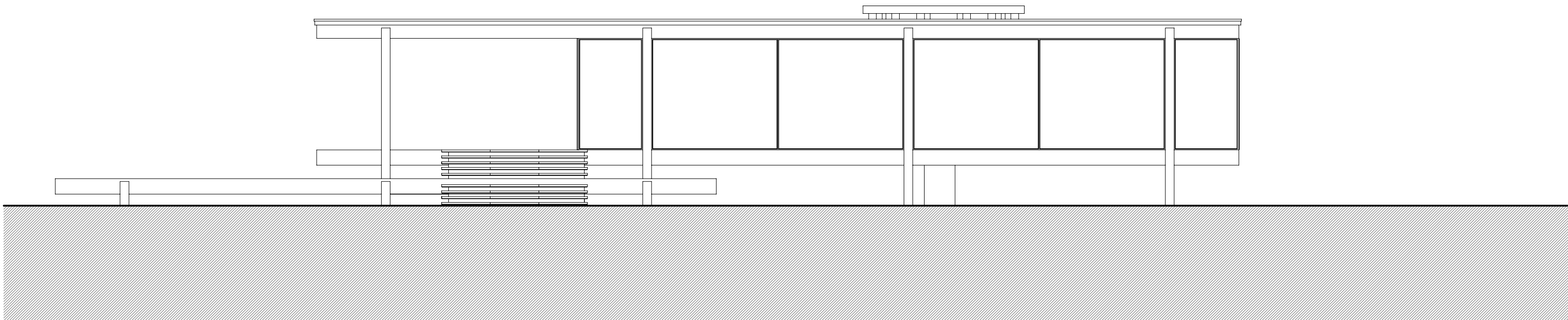
Alçats Sud
