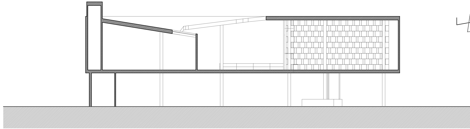
Secció Transversal
