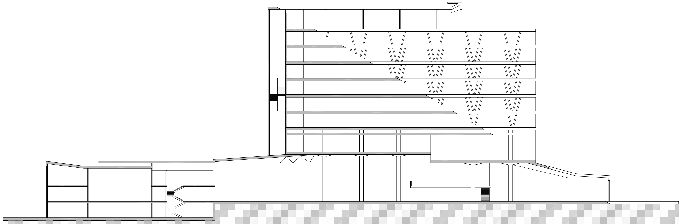
Secció a
