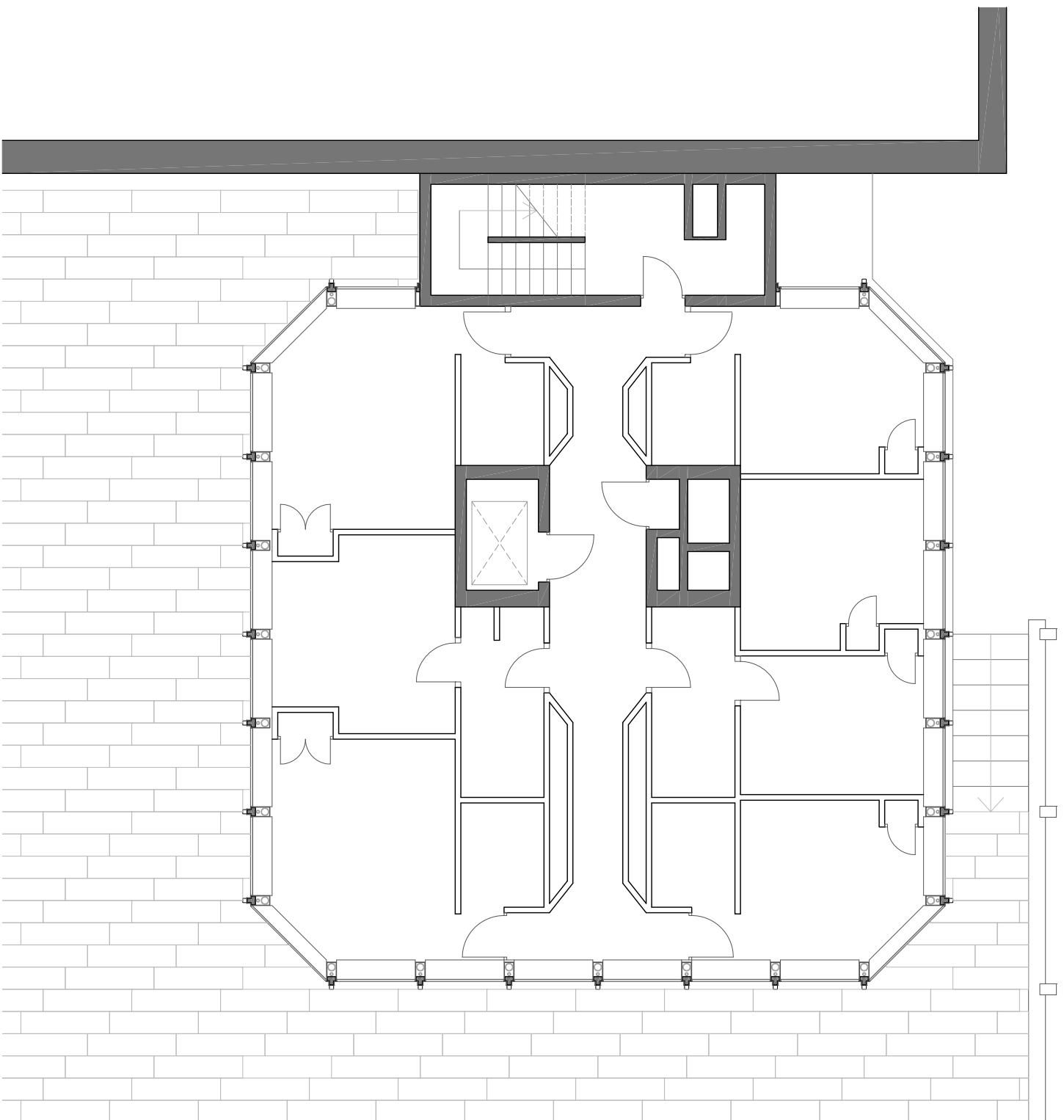
Planta pisos 1-3
