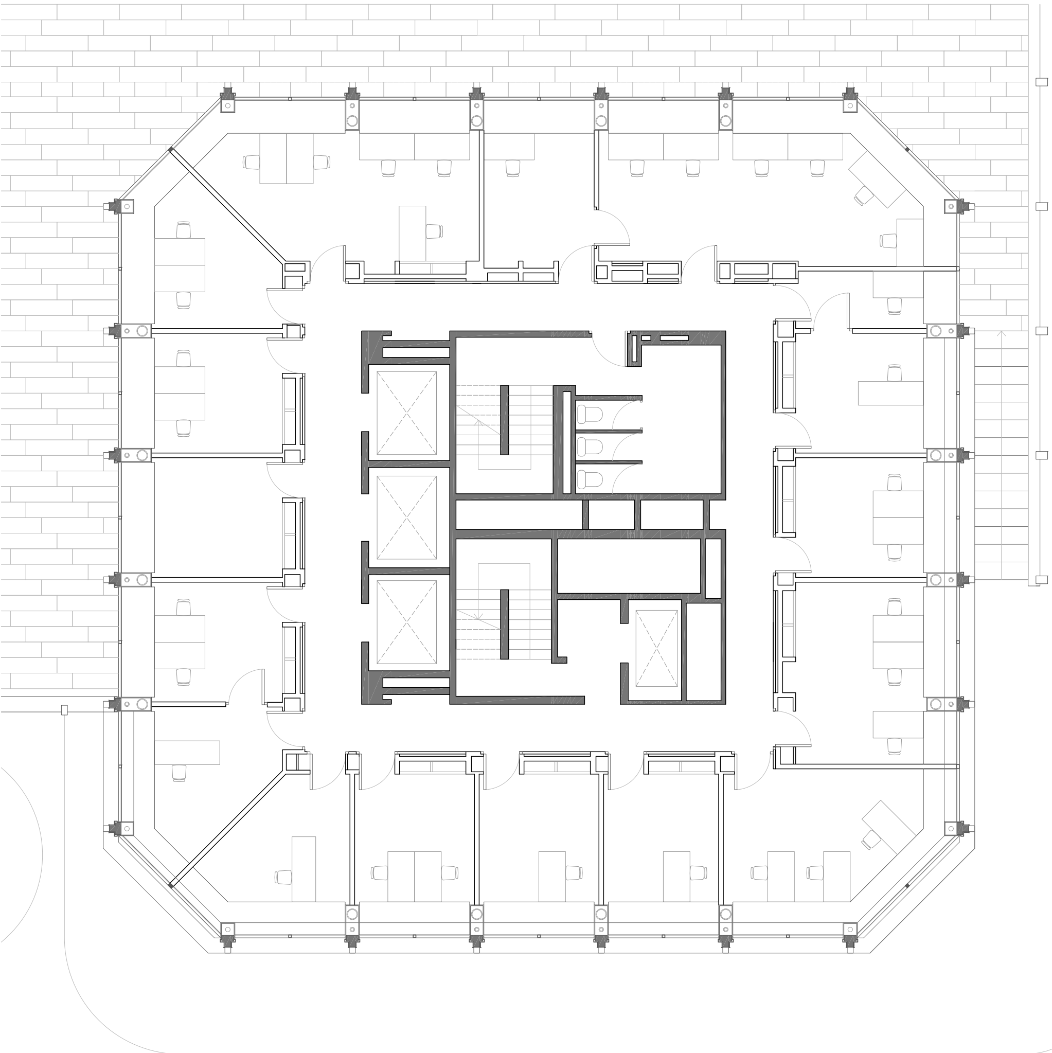
Planta pisos 9-13
