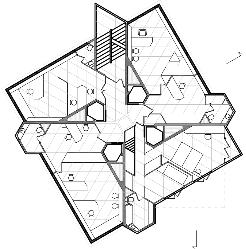
PLANTA TIPUS INFERIOR
